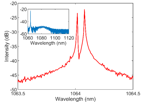
شکل ۳: طیف لیزر نور برگشتی تقویت‌کننده در ۱/۵ وات. در شکل الحاقی، طیف لیزر در محدوده طیفی وسیع‌تری نمایش داده شده است.
