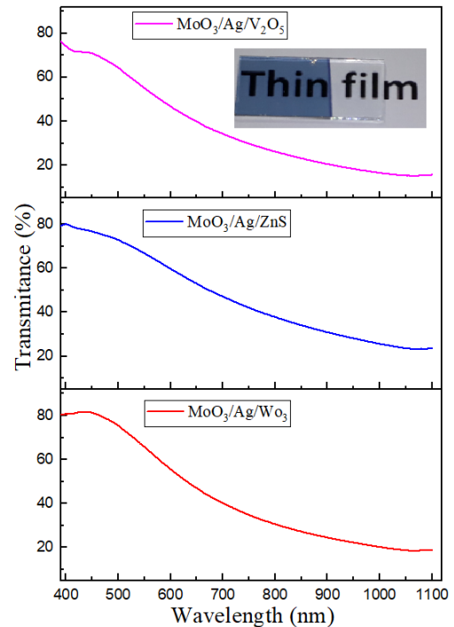
شکل ۲ نمودار تراگسیل اپتیکی ساختارهای ساخته شده و شفافیت سه لایه ای رسانای ساخته شده در آزمایشگاه
