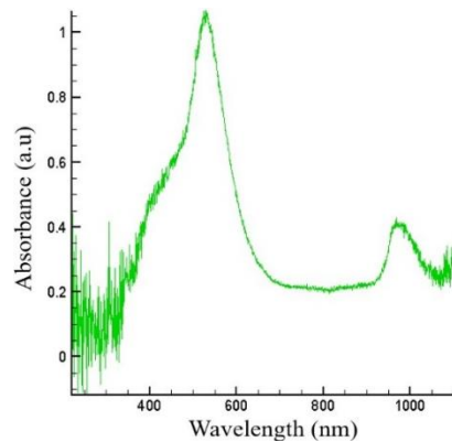
شکل ۱: طیف جذب پلاسمونی نانوذرات طلا ۵۰ نانومتری
