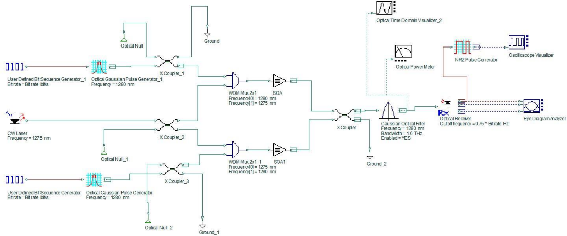
شکل ۱: نمای کلی یک گیت XOR با استفاده از تقویت کننده نوری نیمه هادی و تداخل سنج ماخ زندر.
