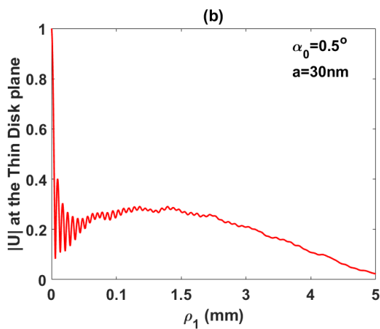
شکل ۲: پروفایل عرضی مد غالب رزوناتور را نشان می‌دهد که بر حسب پارامتر هایپربولید خیلی کوچک رسم شده است.
