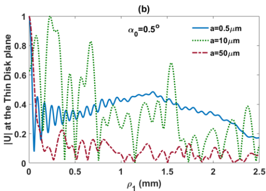
شکل ۳: پروفایل عرضی مد غالب رزوناتور را نشان می‌دهد که بر حسب تغییرات پارامتر هایپربولید رسم شده است.
