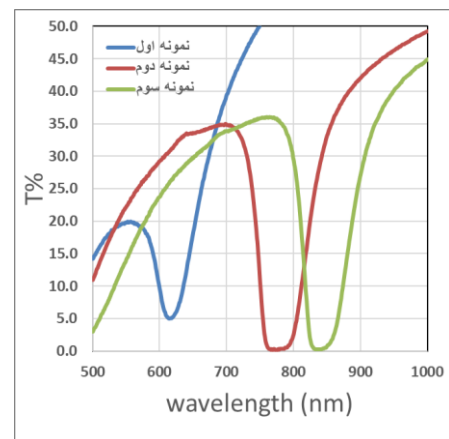
شکل-۳: طیف عبوری از بلورهای فوتونی اوپال سه نمونه ساخته شده در این کار.
