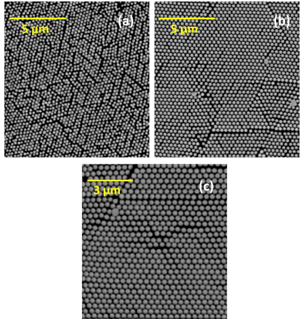
شکل ۲: تصویر SEM از میکرو ذرات پلیمری، شکل (a) مربوط به نمونه اول، شکل (b) مربوط به نمونه دوم و شکل (c) مربوط به نمونه سوم.
