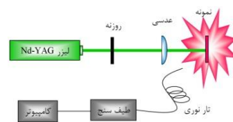
شکل ۲: طرح‌واره‌ی از چیدمان وسایل آزمایش.
