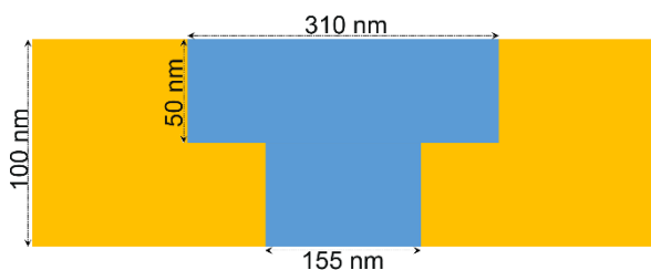
شکل ۱: شمای ساده‌ای از ساختار یک لایه‌ی طلا حاوی دو روزنه- ی استوانه‌ای تو در تو با شعاع‌های ۷۷٫۵ و ۱۵۵ نانومتر
