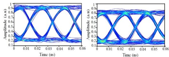
شکل ۵: نمودارهای چشمی 50\text{ Gb/s} . (الف) دامنه 2/3\text{ Vpp} و بایاس معکوس 2\text{ V} . (ب) دامنه 0.7\text{ Vpp} و بایاس معکوس 4\text{ V} .
