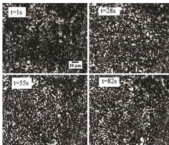
شکل ۲: الگوی لک و سپس حاصل از تفکیک فازی در توده لیپیدی دولایه، با غلظت کلسترول ۲۰٪؛ که تحولات لک و سپس ها را با زمان نشان می دهد.
