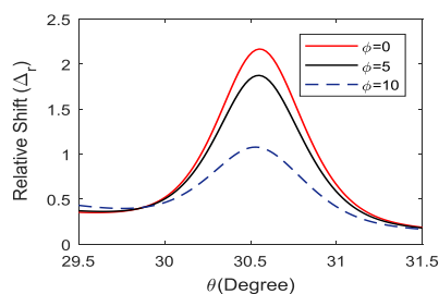
شکل ۳: جابجایی عرضی باریکه بازتابی از فصل مشترک فراماده هایپربولیک و هوا بر حسب زاویه فرودی در \varphi=0^\circ ، \varphi=5^\circ و \varphi=10^\circ که به ترتیب در فرکانس‌های f=7.87THz ، f=8.16THz و f=10THz رسم شده است.
