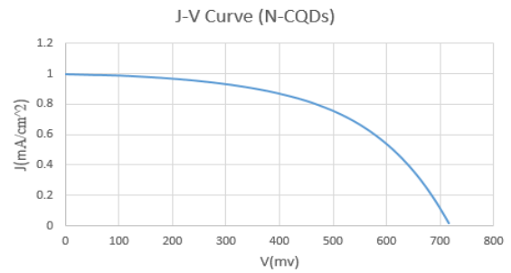
شکل ۵: منحنی چگالی جریان - ولتاژ مربوط به سلول خورشیدی حساس شده به N-CQDs سنتز شده
