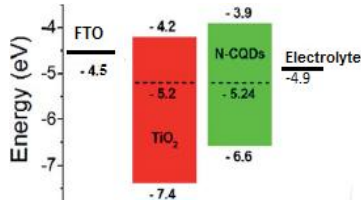
شکل ۶: نمایی از همخوانی ترازهای انرژی لایه‌های سلول [۳]
