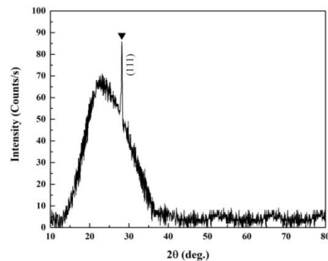
شکل ۱: الگوی پراش پرتو ایکس نقاط کوانتومی سیلیکون.
