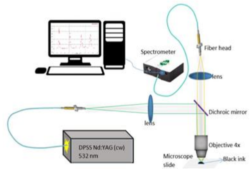
شکل ۱: چیدمان آزمایش اندازه‌گیری جابه‌جایی رامان جوهر.
