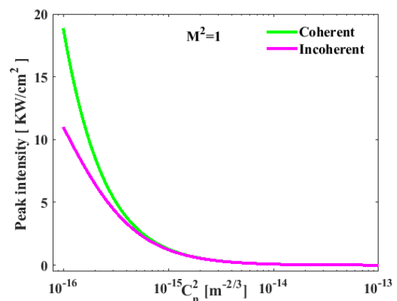
شکل ۲: مقایسه قله شدت در روش همدوس و ناهمدوس.
