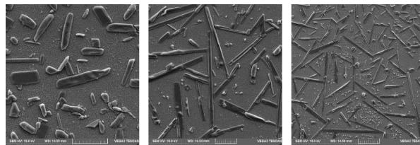
شکل ۴: تصویر SEM از لایه‌ی نازک اکسید مولیبدن رشد یافته با استفاده از روش الکتروشیمی. خط مقیاس به ترتیب از سمت چپ، ۱۰، ۱۰، ۲۰ میکرون است.
