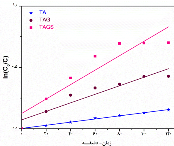
شکل ۲: نمودار ضریب k_{app} ایزوپروپیل تیتانیا و نانوکامپوزیت‌های تولید شده.
