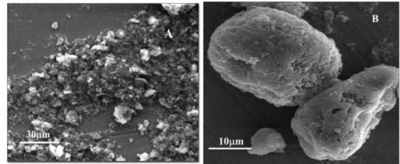
شکل ۱: تصاویر میکروسکوپ الکترونی روبشی از ذرات کربن نیتريد.
