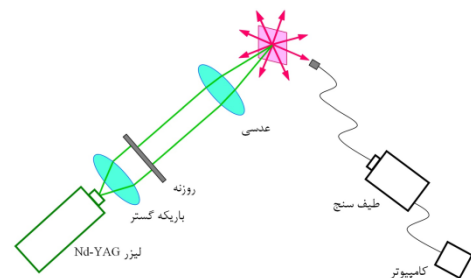
شکل ۲: طرح‌واره‌ی از چیدمان آزمایش.
