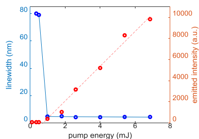
شکل ۴: منحنی شدت بیشینه و پهناي قله‌ی تابشی بر حسب انرژی هر پالس دمشی.
