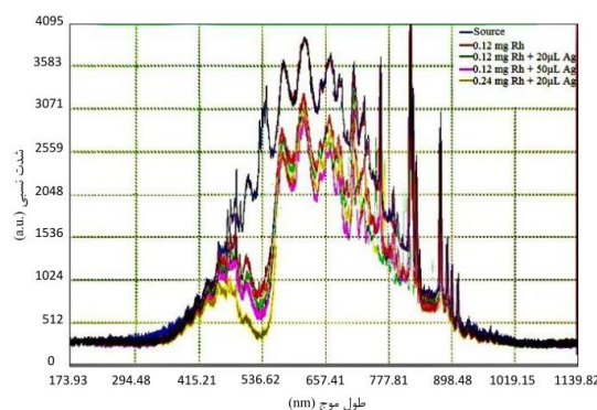
شکل ۴: طیف عبوری از فیلم‌های تهیه شده با جوهر نانو ذرات نقره
