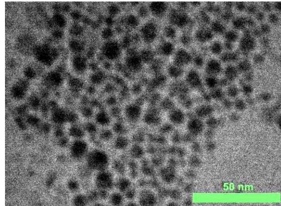
شکل ۱: تصویر TEM جوهر نانو ذرات نقره
