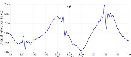
شکل ۳: نمایش شکل خط تشدید فانو در شکاف هوا (الف) ۵۰ نانومتر (ب) ۱۵۰ نانومتر (ج) ۲۵۰ نانومتر (د) ۳۵۰ نانومتر (ه) ۴۵۰ نانومتر (و) ۵۵۰ نانومتر
