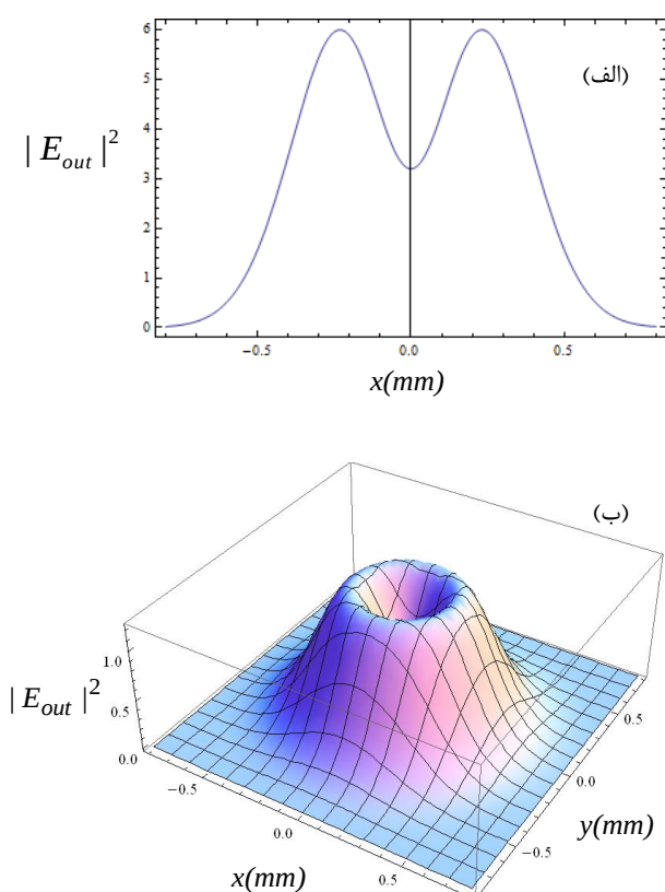
شکل ۲: شدت میدان خروجی تشدیدگر تخت-تخت که بعد از ده بار رفت و برگشت (الف) شکل دو بعدی و (ب) شکل ۳ بعدی میدان. در اینجا و در شکل‌های بعد |E_{out}|^2 برحسب واحد اختیاری رسم شده است.
