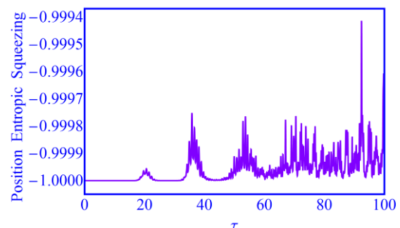
شکل ۴: چلانگی آنتروپی برحسب زمان مشخصه \tau = gt در حالت تشدید بازای |\alpha|^2 = 10 = |\beta|^2 ، \delta = 0.1 ، \gamma = 1 و \chi = 0 .
