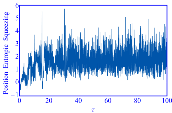
شکل ۳: چلانگی آنتروپی برحسب زمان مشخصه \tau = gt در حالت تشدید بازای |\alpha|^2 = 10 = |\beta|^2 ، \delta = 0.1 ، \gamma = 1 و \chi = 0.4 .
