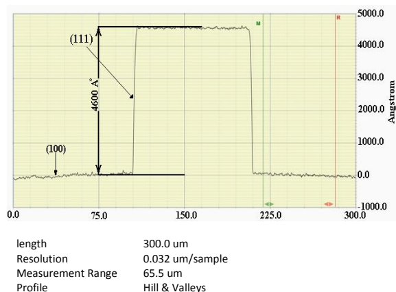
شکل ۳- نمودار پروفایل سطحی ویفر (۱۰۰) GaAs سونش شده
