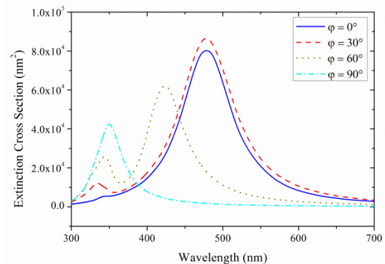
شکل ۳: مدهای طولی ( f = 0 )، عرضی ( f = 90 ) و هیبریدی ( 0 < f < 90 ) برانگیخته شده به ازای زاویه قطبی q = 90 برای بیضیگونی با a = b = 30 nm و c = 60 nm.
