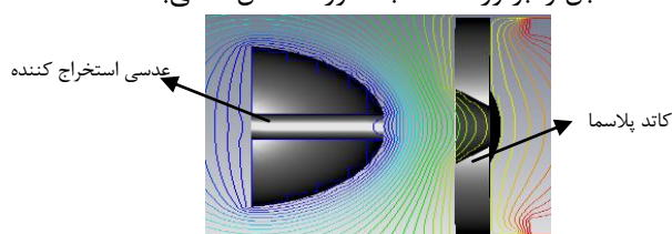
شکل ۲: سیستم استخراج طراحی شده
