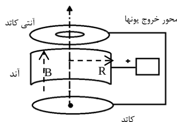
شکل ۱: طرح واره چشمه پنینگ
