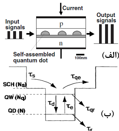
شکل ۳: (الف) ساختار تقویت‌کننده نوری نیم‌رسانا نقطه کوانتومی [۱] (ب) ترازهای انرژی QD در نوار رسانش تقویت‌کننده [۴]
