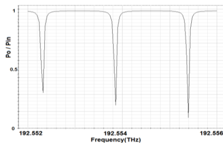
شکل ۷ پاسخ فرکانسی تشدیدگر با شعاع ۳cm- ضریب تزویج ۰,۰۵db- تلفات ۰,۰۵db/cm
