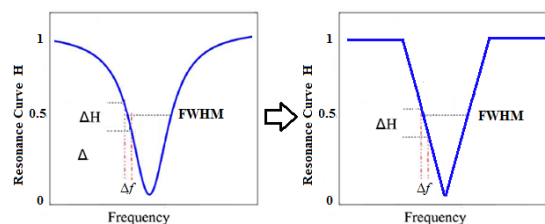
شکل ۸ تقریب خطی سازی برای پاسخ فرکانسی تشدیدگر حلقوی
