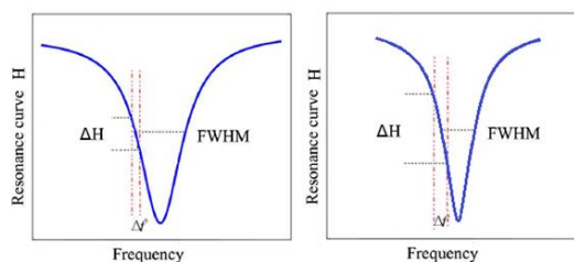
شکل ۷ نمودار پاسخ فرکانسی برای دو تشدیدگر با FWHM متفاوت
