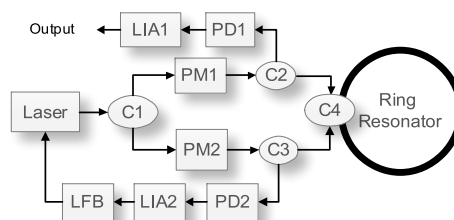
شکل ۱ بلوک دیاگرام کلی ژیروسکوپ نوری تشدیدی
