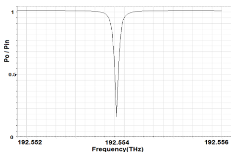
شکل ۶ پاسخ فرکانسی تشدیدگر با شعاع ۱,۵cm- ضریب تزویج ۰,۰۵db- تلفات ۰,۰۵db/cm
