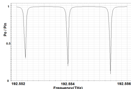
شکل ۹ پاسخ فرکانسی تشدیدگر با شعاع ۳cm- ضریب تزویج ۰,۰۵db- تلفات ۰,۰۵db/cm
