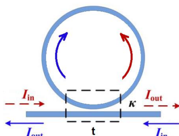
شکل ۲ ساختار تشدیدگر حلقوی
