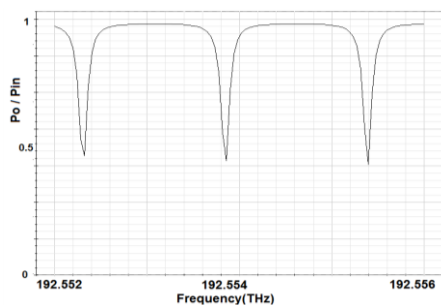
شکل ۱۰ پاسخ فرکانسی تشدیدگر با شعاع ۳cm- ضریب تزویج ۰,۰۵db- تلفات ۰,۱db/cm
