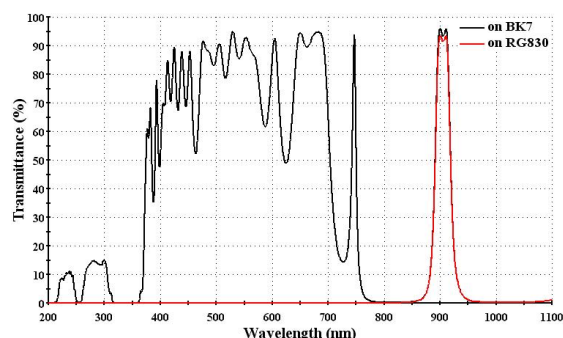
شکل ۱: طیف تراگیل شبیه سازی شده ی پالایه ی طراحی شده بر روی بستره های BK۷ و RG۸۳۰.
