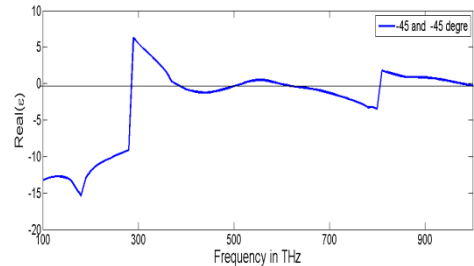
شکل ۶: طیف ثابت‌دی الکتریک موثر ساختار جاذب طراحی شده
