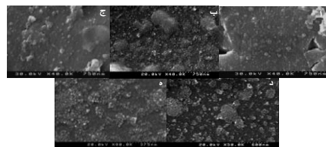
شکل ۳: تصویر SEM از پنج نمونه سنتز شده در میدان مغناطیسی با شدت: (آ) ۰، (ب) ۰/۰۱، (ج) ۰/۰۴، (د) ۰/۰۹، (ه) ۰/۱۳ تسلا
