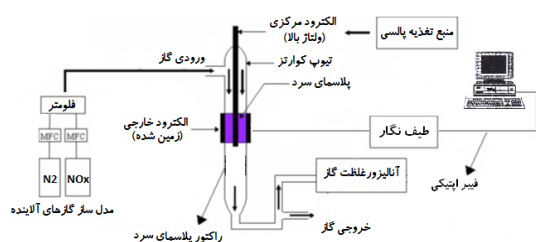
شکل ۱: چیدمان آزمایش
