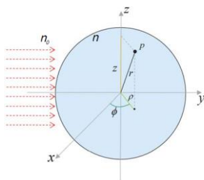
شکل ۳: گرادیان ضریب شکست و دما در اطراف ذره گرم شده
