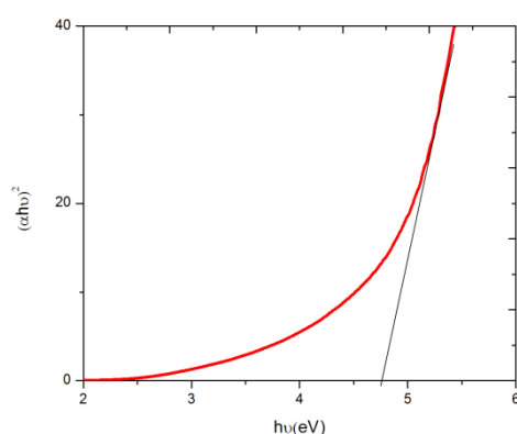
شکل ۲-ب (۳): گاف انرژی اکسید کادمیم ۱٪ آلاینده شده با آهن
