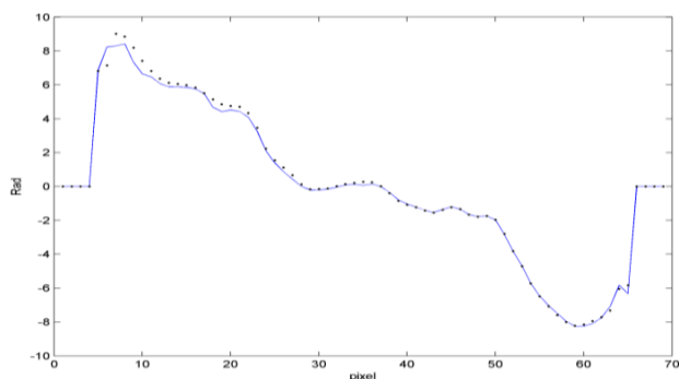
شکل ۸: نمودار خط‌چین نشان دهنده سطر ۳۰ مربوط به اختلاف فاز بازسازی شده (اختلاف شکل‌های ۶ و ۷) و نمودار توپر اختلاف فاز دو باریکه که با روش انتقال فاز به دست آمده است. محور افقی شماره پیکسلها و محور عمودی بر حسب رادیان می‌باشد.
