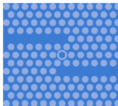
شکل ۱: ساختار حسگر فشار با a=440 \text{ nm} و شعاع حفره‌های هوای r=158/4 ، شعاع خارجی و داخلی میکروکاواک به کارگرفته شده به ترتیب ۲۴۲ nm و ۱۴۸ nm می‌باشند.
