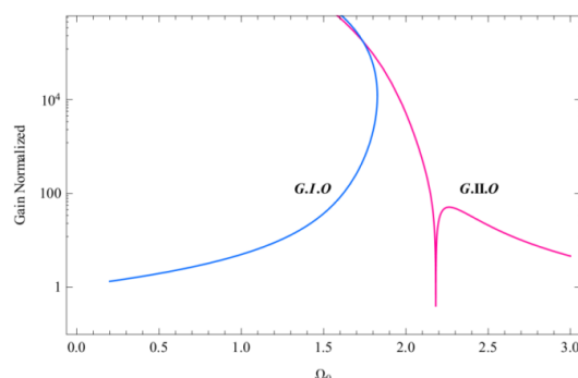
شکل ۵: نمودار بهره بهنجار بر حسب فرکانس بهنجار میدان مغناطیسی محوری برای \gamma = 8 ، \Omega_L = 0.05 و \omega_b = 0.1 .
