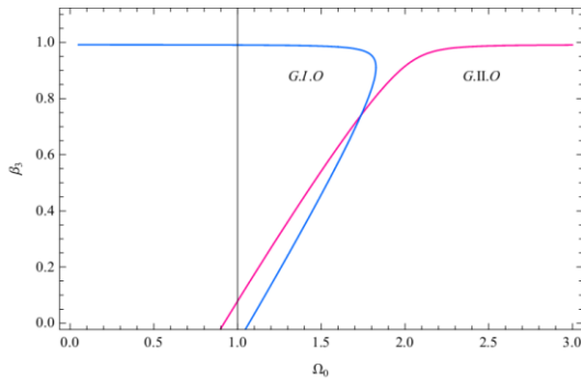
شکل ۳: نمودار سرعت محوری بهنجار به صورت تابعی از فرکانس بهنجار میدان مغناطیسی راهنمای محوری برای مدارهای گروه های I و II. پارامترهای انتخاب شده عبارتند از \gamma = 8 ، \Omega_L = 0.05 و \omega_b = 0.1 .
