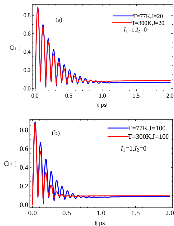
شکل ۲: تحول زمانی جمعیت درهم‌تنیدگی دو جایگاه مولکولی در دو دمای T=77K و 300K به ازای (a) جفت‌شدگی الکترونی ضعیف و (b) جفت‌شدگی قوی الکترونی مولکول‌های رنگدانه
