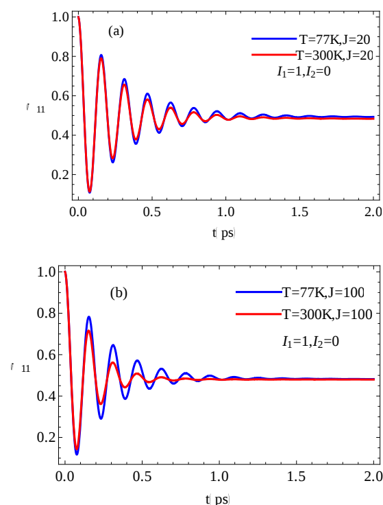
شکل ۳: تحول زمانی جمعیت جایگاه اول در دو دمای T=77K و 300K به ازای (a) جفت‌شدگی الکترونی ضعیف و (b) جفت‌شدگی قوی الکترونی مولکول‌های رنگدانه
