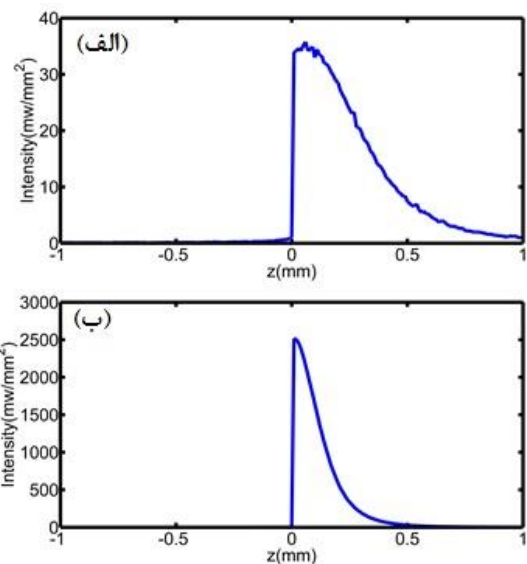
شکل ۳: شدت بر حسب ارتفاع بر روی محور فیبرنوری با قطر (الف): 200 \mu\text{m} و (ب): 10 \mu\text{m} (پایین)
