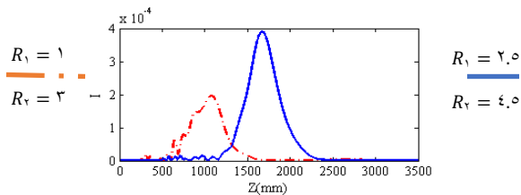
شکل ۳- شدت در امتداد محور اپتیکی
