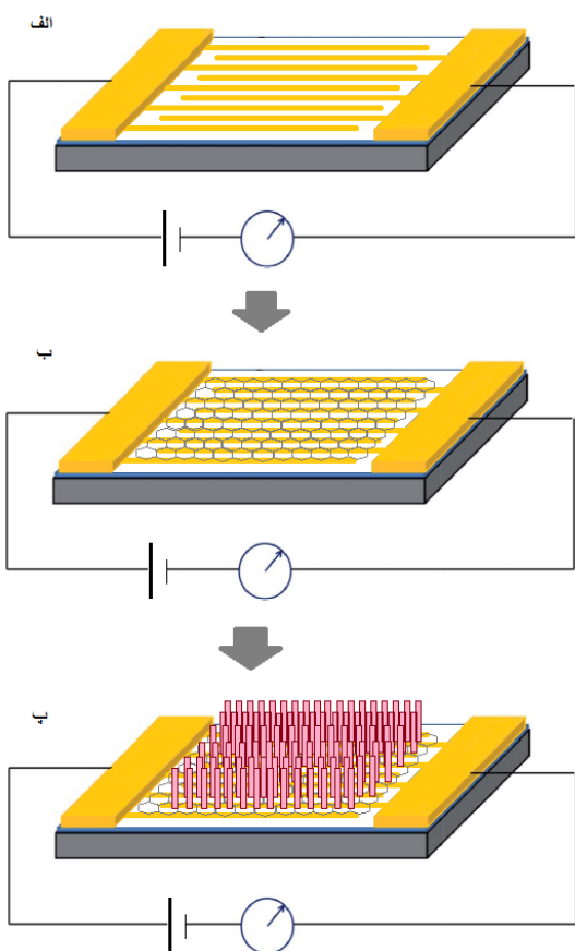
شکل ۱: مراحل ساخت آشکارساز فرابنفش با استفاده از ساختار \text{ZnO NWS-RGO} (الف) لیتوگرافی الکترودهای طلا بر روی بستر شیشه (ب) قراردادن صفحه اکسید گرافن بر روی الکترودها (پ) رشد نانو سیم های \text{ZnO} بر روی گرافن
