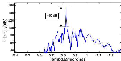
شکل ۴. طیف سیگنال خروجی لیزر وکسل کریستال نوری در حالت استفاده از روزنه اکسید با R_o = 0.6 \mu\text{m}
