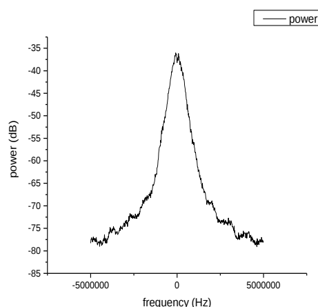
شکل ۴: طیف تداخل با پهنای طیف 3dB، 233KHz در محدوده فرکانسی 5MHz (روش مستقیم)
