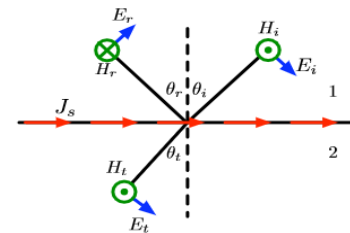
شکل ۲- میدان های الکتریکی و مغناطیسی در قطبش P
