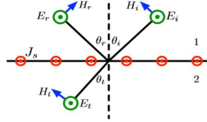
شکل ۱- میدان های الکتریکی و مغناطیسی در قطبش S
