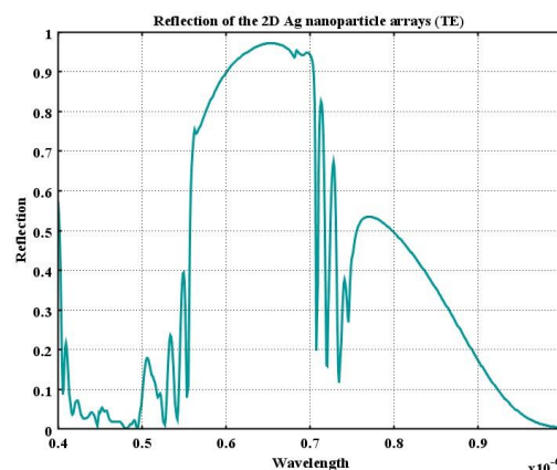
شکل ۷: طیف انعکاسی نمونه بلور فوتونی فلزی ساخته‌شده از قالب پلی استایرن. باند گاف فوتونی کامل در بازه طیفی ۷۰۰-۵۷۰ nm تشکیل شده است.
