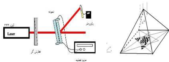
شکل ۲: منشور هرمی
