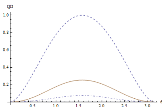
شکل ۱. تغییرات ناهم‌خوانی کوانتومی تحت کانال واقطبش تعمیم یافته نسبت به \theta . منحنی خط-چین به ازای \lambda=1 ، خط تیره به ازای \lambda=0 ، و نقطه خط-چین به ازای \lambda=1/2 رسم شده است.
