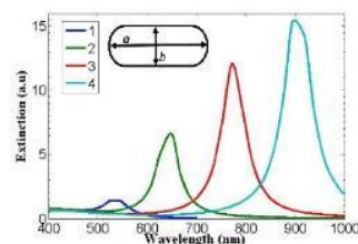
شکل ۶: سطح مقطع خاموشی برای نانومیله‌های طلا با شعاع مؤثر ۳۰ nm و نسبت ابعاد (a/b) مختلف.
