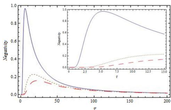
شکل ۲: نمودار درهمتیدگی بر حسب \tau برای سه مقدار مختلف \bar{\chi} : \bar{\chi} = 0.7 (خط ممتد)، \bar{\chi} = 0.9 (نقطه چین) و \bar{\chi} = 1 (خط چین). شکل الحاقی رفتار درهمتیدگی در دمای های کوچک را نشان می‌دهد.
