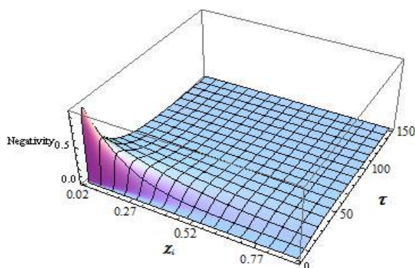
شکل ۳: نمودار سه بعدی درهمتیدگی براساس دما و عامل غیرخطی خوددکشی.
