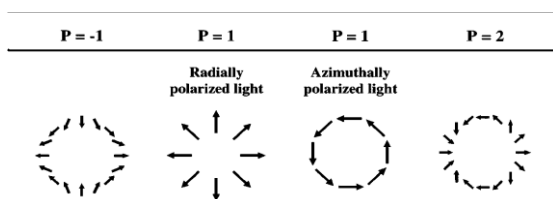
شکل ۱: نمونه‌هایی از نور پلاریزه‌ی خطی با تقارن محوری [۶].
