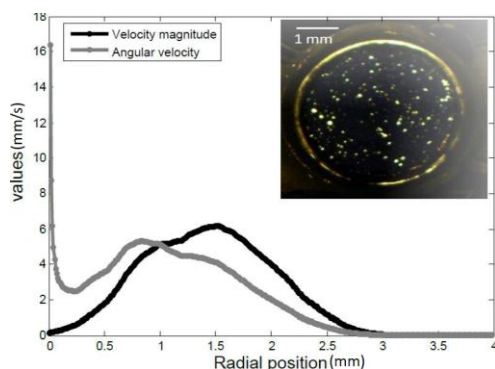
شکل ۴: تغییر سرعت چرخش برحسب تغییر شعاع.
